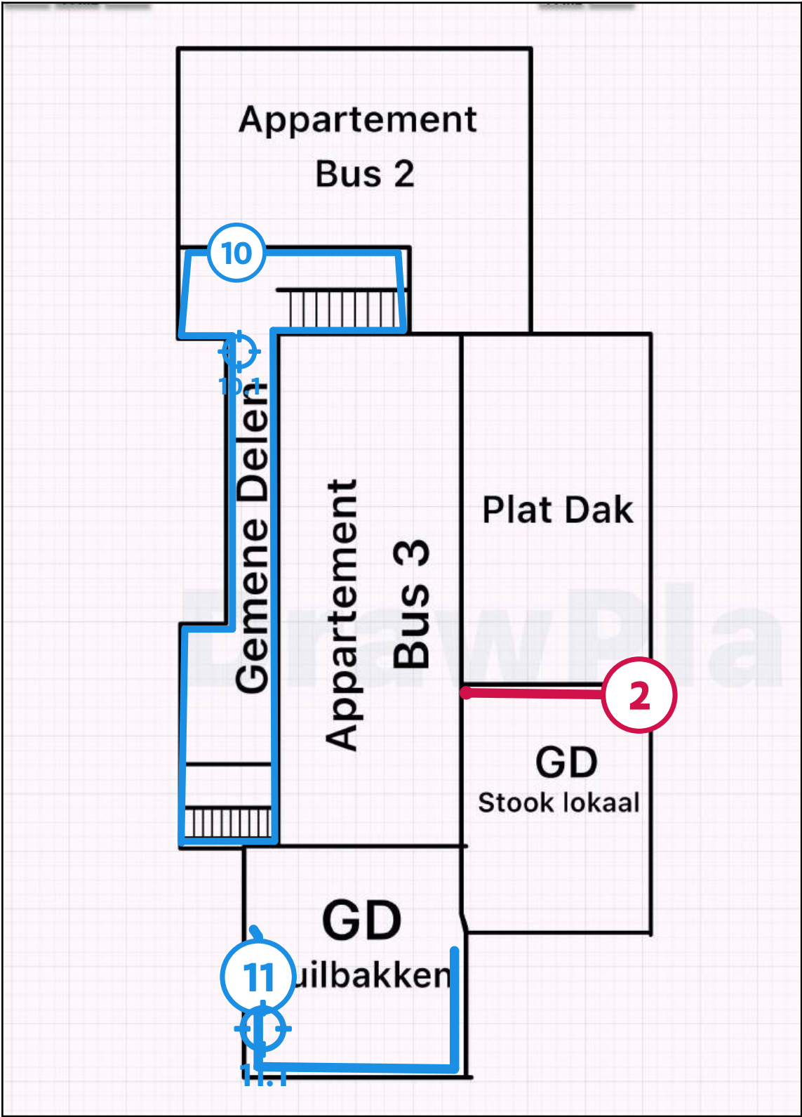
Legende van plan 1.3: 1e verdieping
