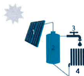
1 Zonnecollector | 2 Zonneboiler 3 Opslagvat voor warm water 4 Radiator
