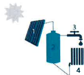
1 De zonnecollector | 2 Opslagvat voor warm water | 3 Sanitair warm water | 4 Aansluiting op de verwarming
