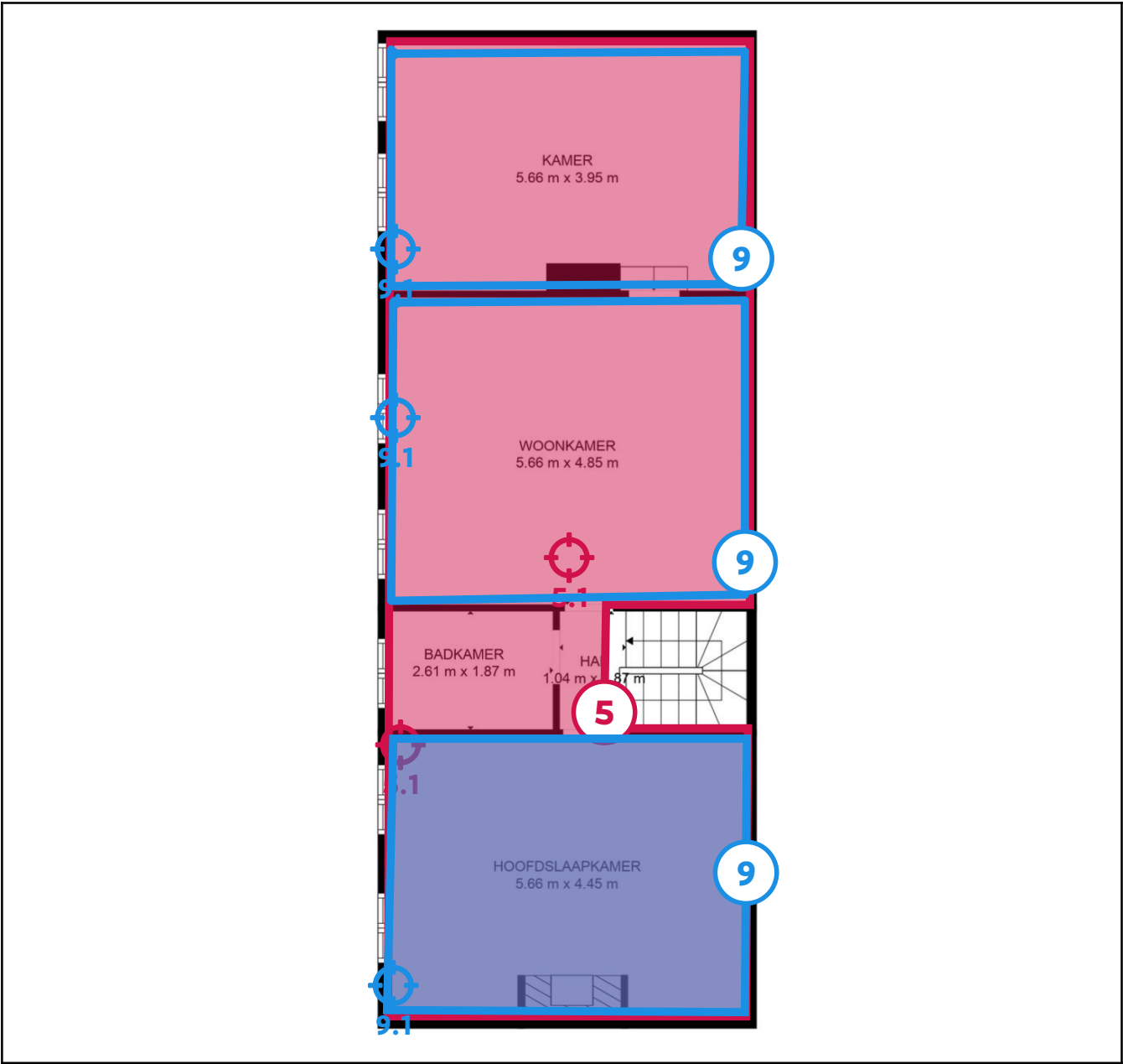
Legende van plan 3.2: Hoofdgebouw - eerste verdieping
