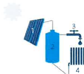
1. Zonnecollector 2. Opslagvat zonnewater 3. Kraan 4. Radiator
