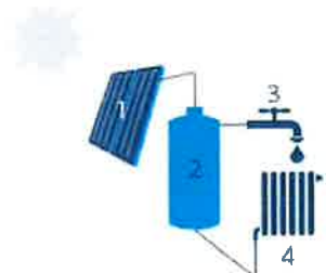
1. Zonnecollector | 2. Opslagvat voor warm water | 3. Tap | 4. Radiator
