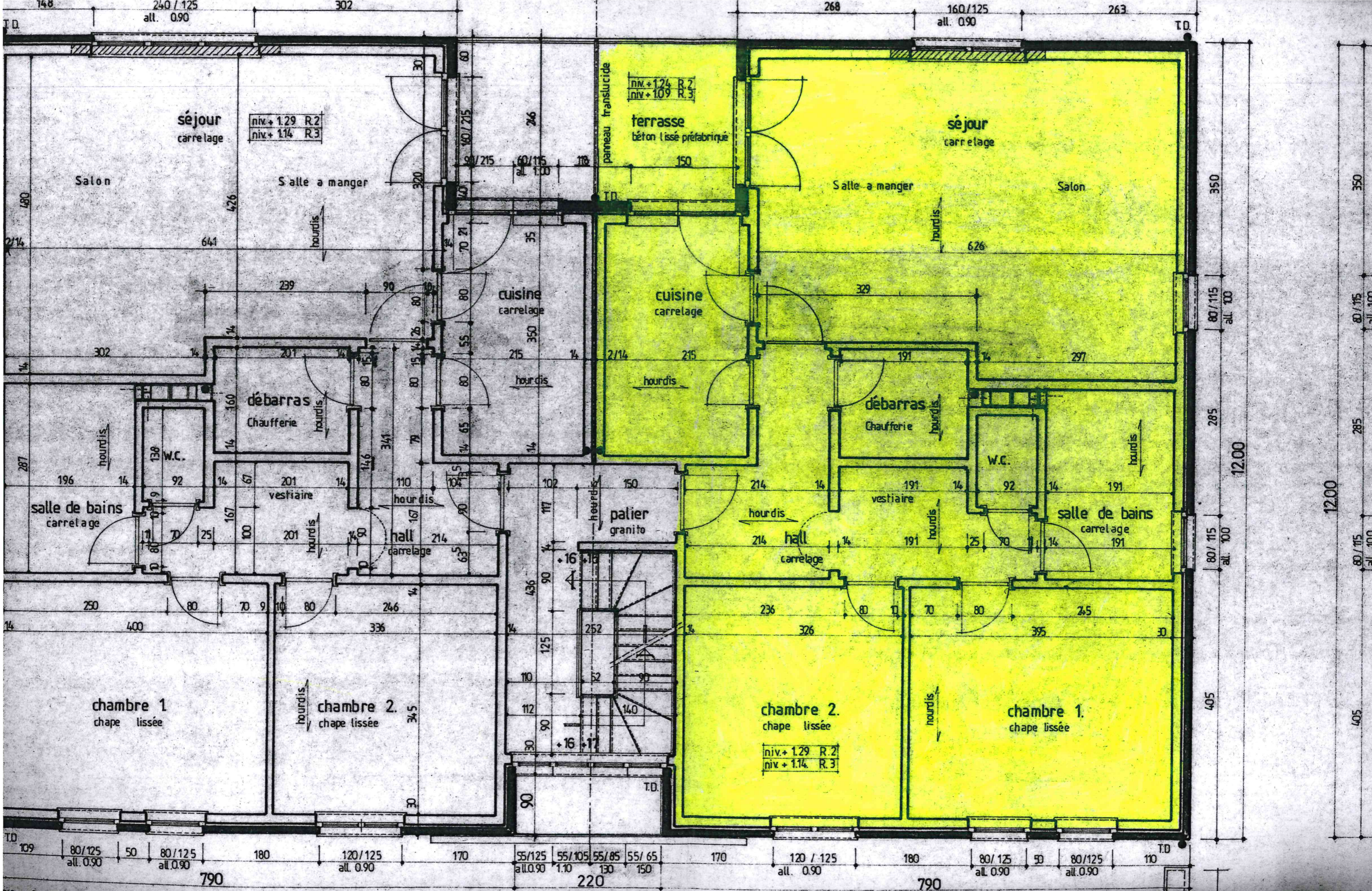
PLAN DU 1er ETAGE - Residences 2 et 3-
