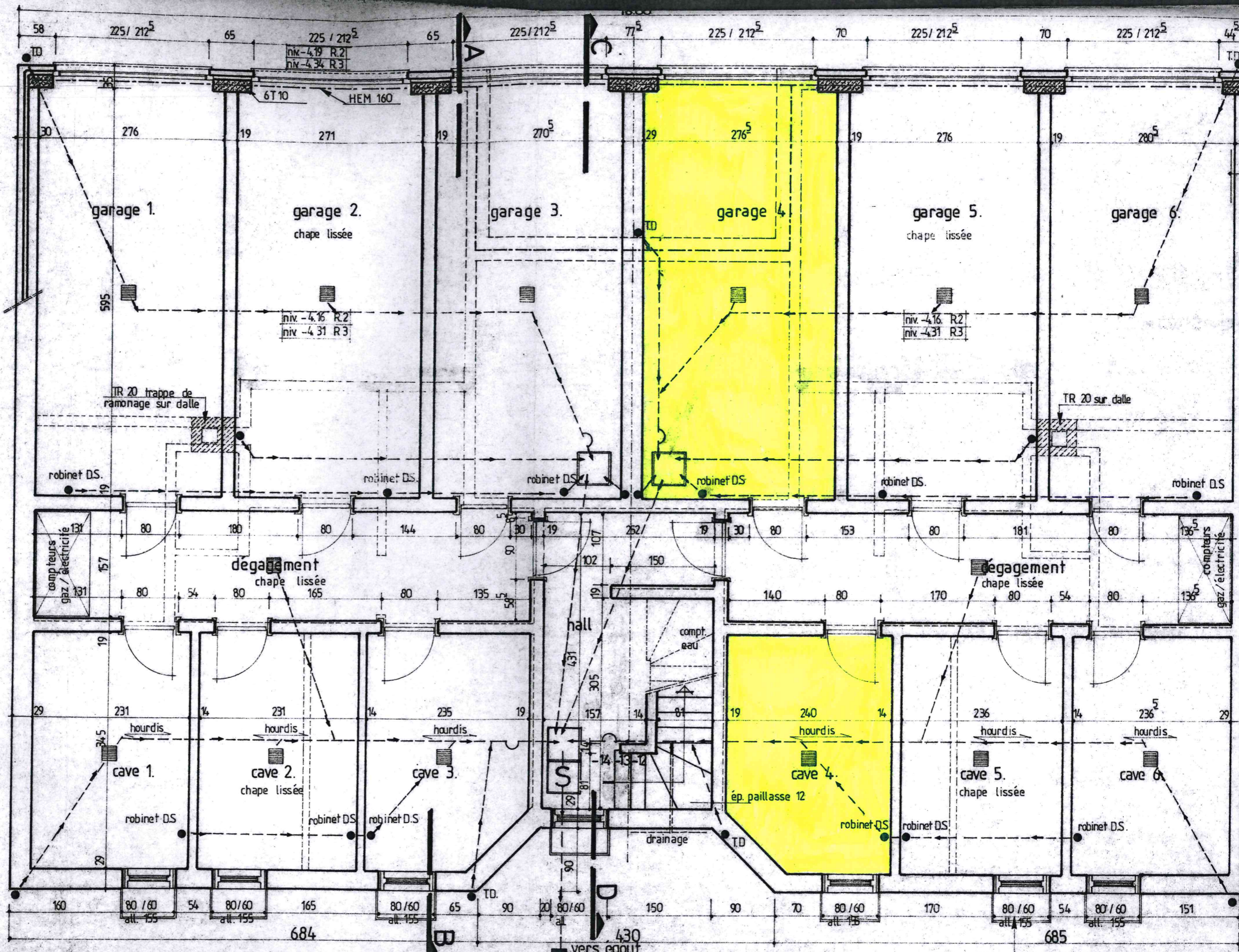
PLAN DES SOUS-SOLS — FONDATIONS — CANALISATIONS
