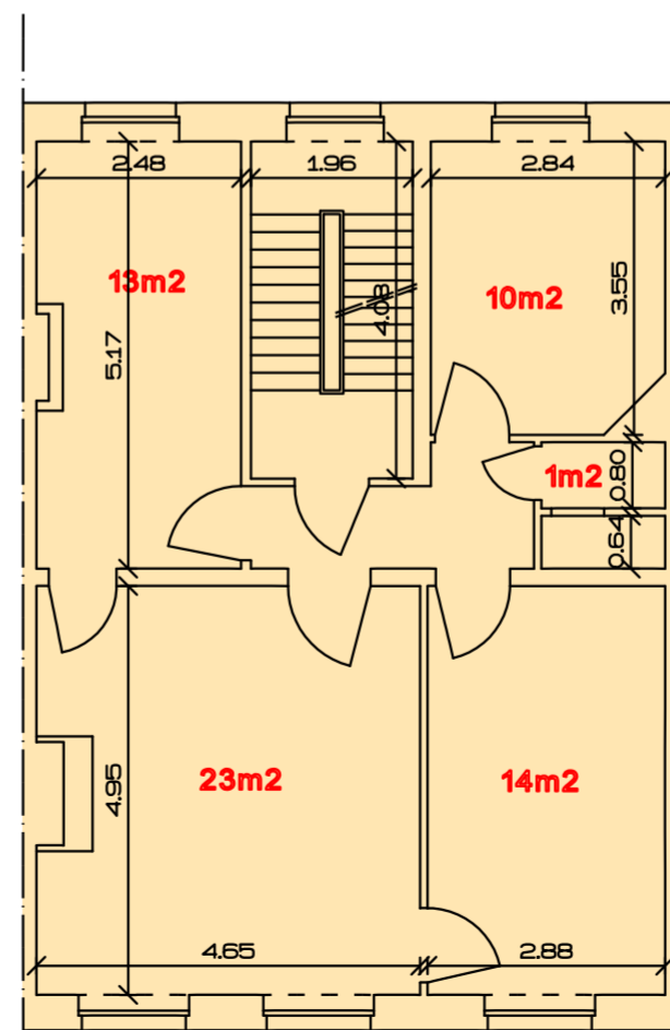
SURF. BRUTE : 89,17 m 2 DEUXIEME ETAGE
