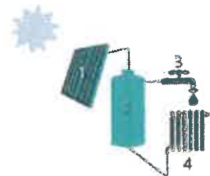
1. Zonnecollector | 2. Opslagvat zonneboiler | 3. Sanitair warm water | 4. Afgifte-element voor ruimteverwarming (opuloneet)
