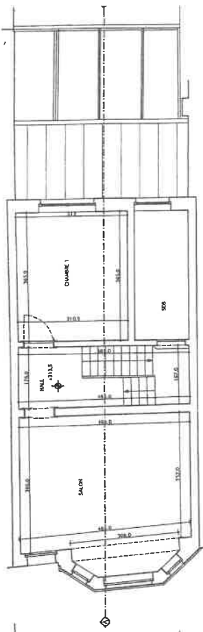
Plan du 1er Etage - 1/100e
