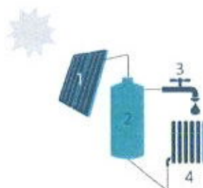
1. Zonnecollector | 2. Opslagvat voor warm water | 3. Sanitair kraanpunt | 4. Radiator
