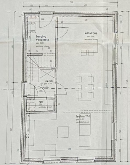
GELJKVLOERS schaal 1/50
