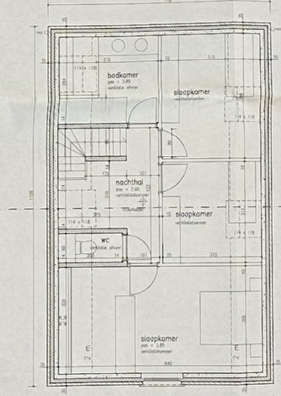
VERDIEPINGSPLAN schaal 1/50
