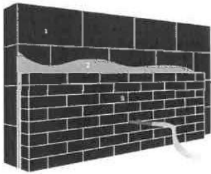
1. Dragende muur | 2. Ingeblazen isolatie | 3. Gevelsteen / gevelbekleding
