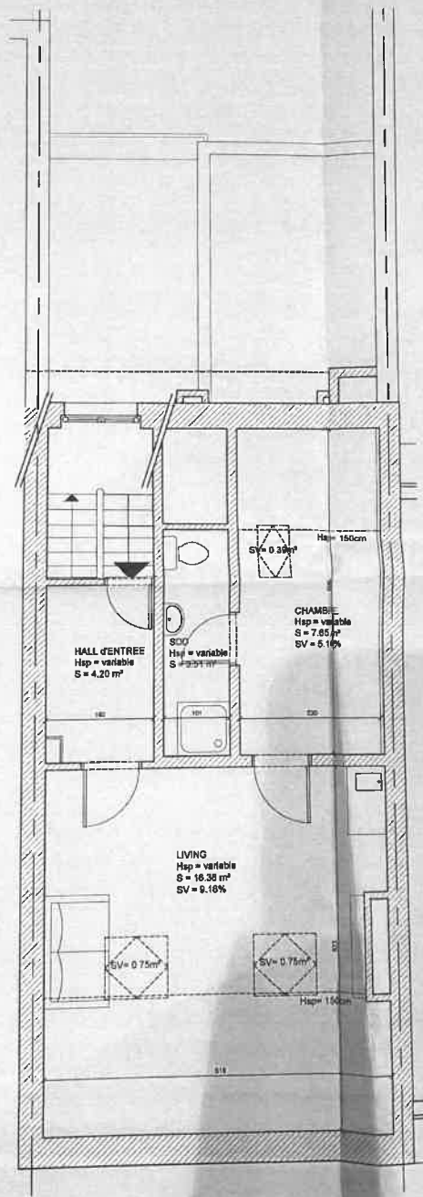
Situation existante - PLAN DES COMBLES
