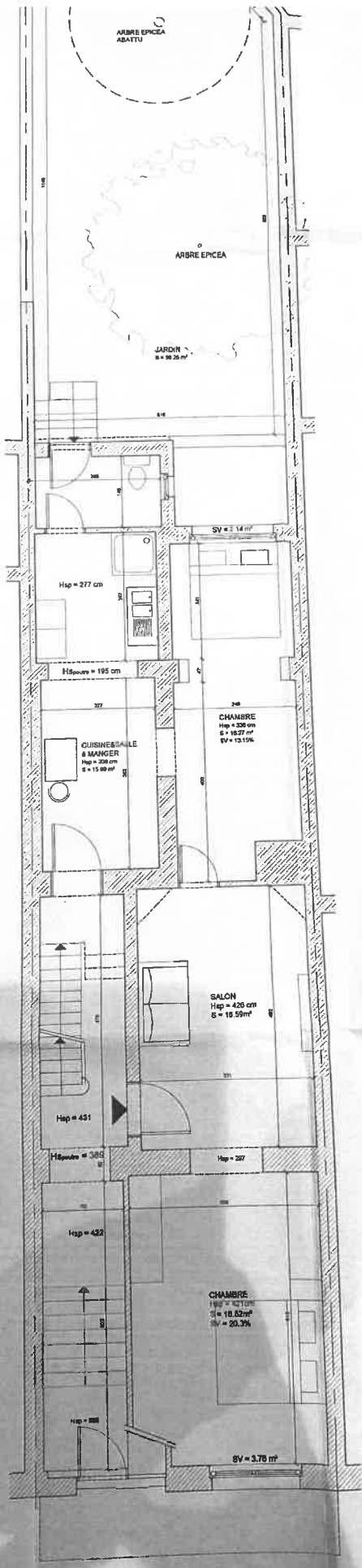
Situation existante - PLAN DE REZ-DE-CHAUSSEE
