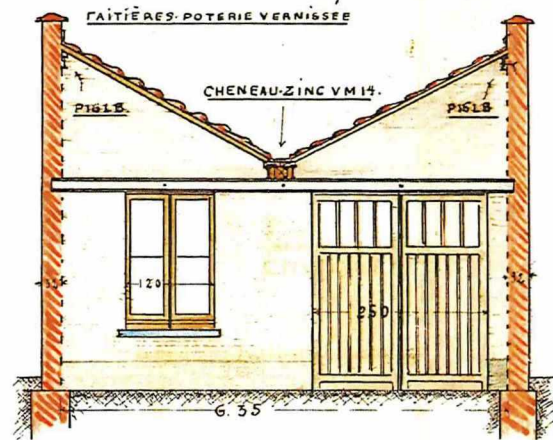
MAGASIN - ÉLEVATION
