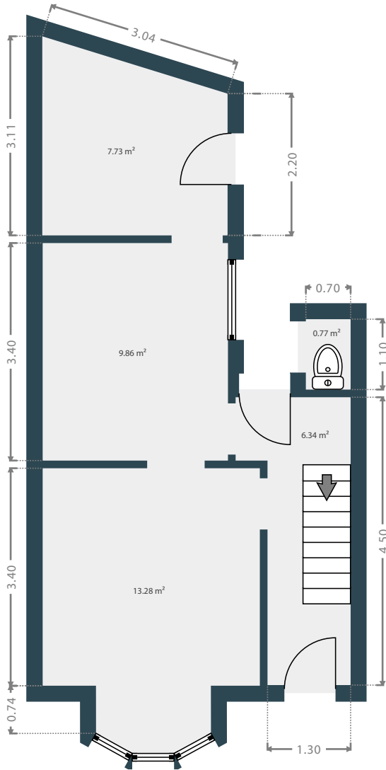
Rez-de-chaussée
