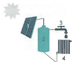
1. Zonnecollector | 2. Opslagvat zonneboiler | 3. Sanitair warm water | 4. Afgiftesysteem voor ruimteverwarming (optioneel)
