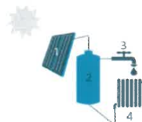
1 Zonnecollector | 2 Opslagvat warmwater | 3 Sanitair warm water | 4 Afgeefelement voor ruimtewarmte
