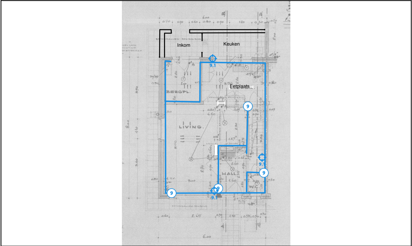
Legende van plan 1.9: Plan gelijkvloers
