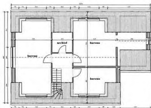
dakverdieping (nieuw / schaal : 1 - 50)
