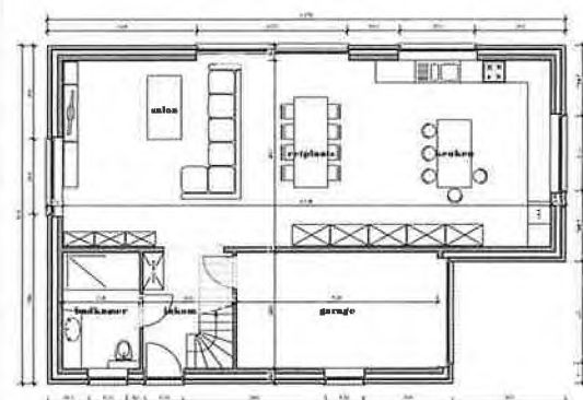
gelijkvloers (nieuw / schaal : 1 - 50)
