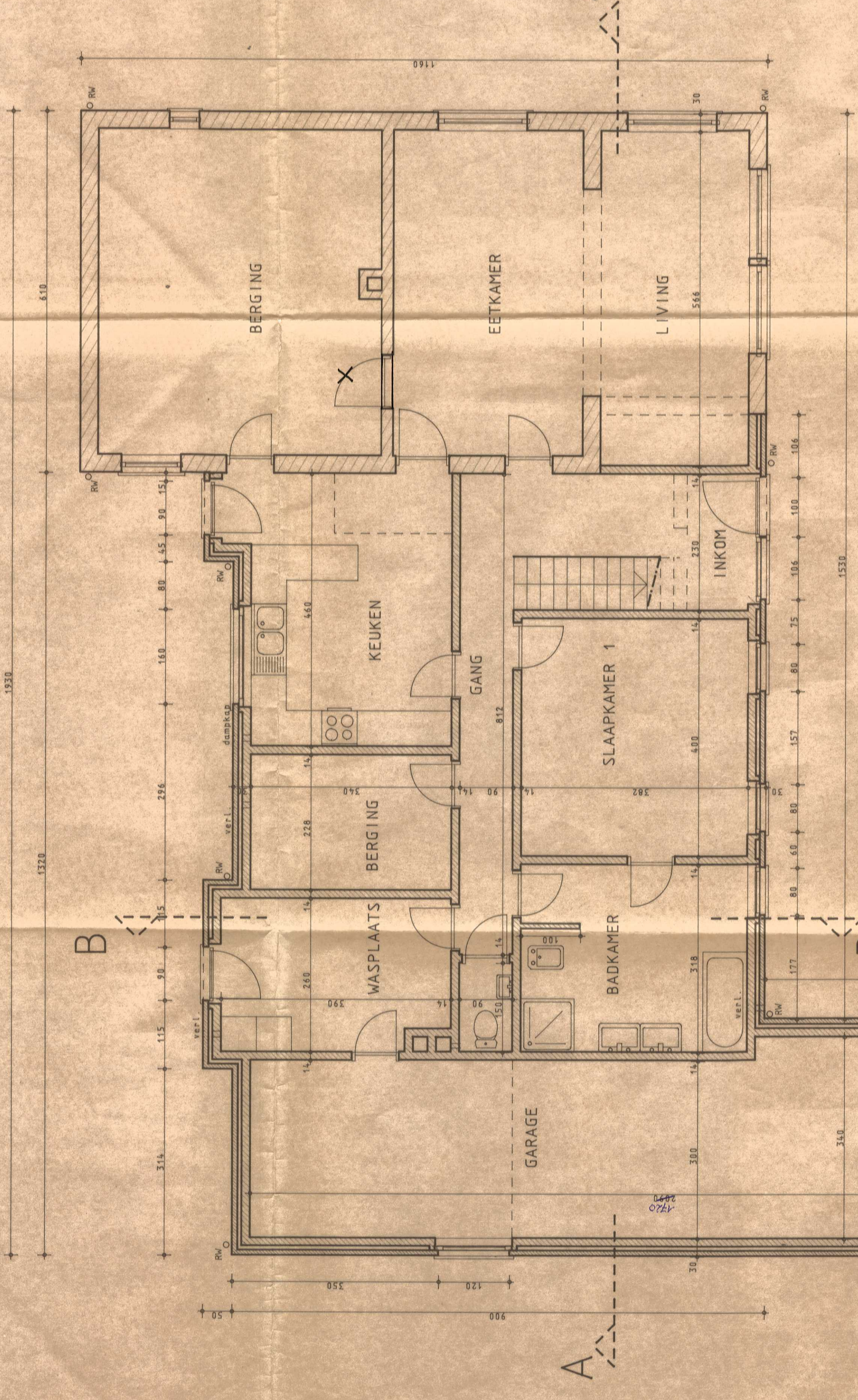
GRONDPLAN
