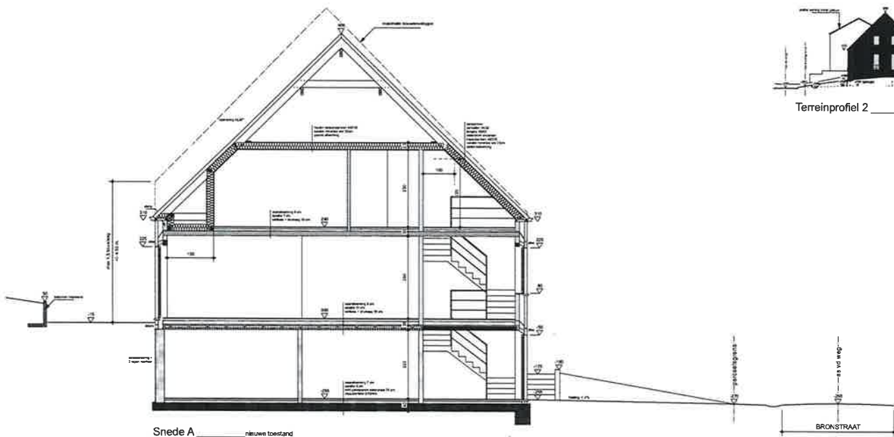
Sneede A _____ nieuwe toestand
