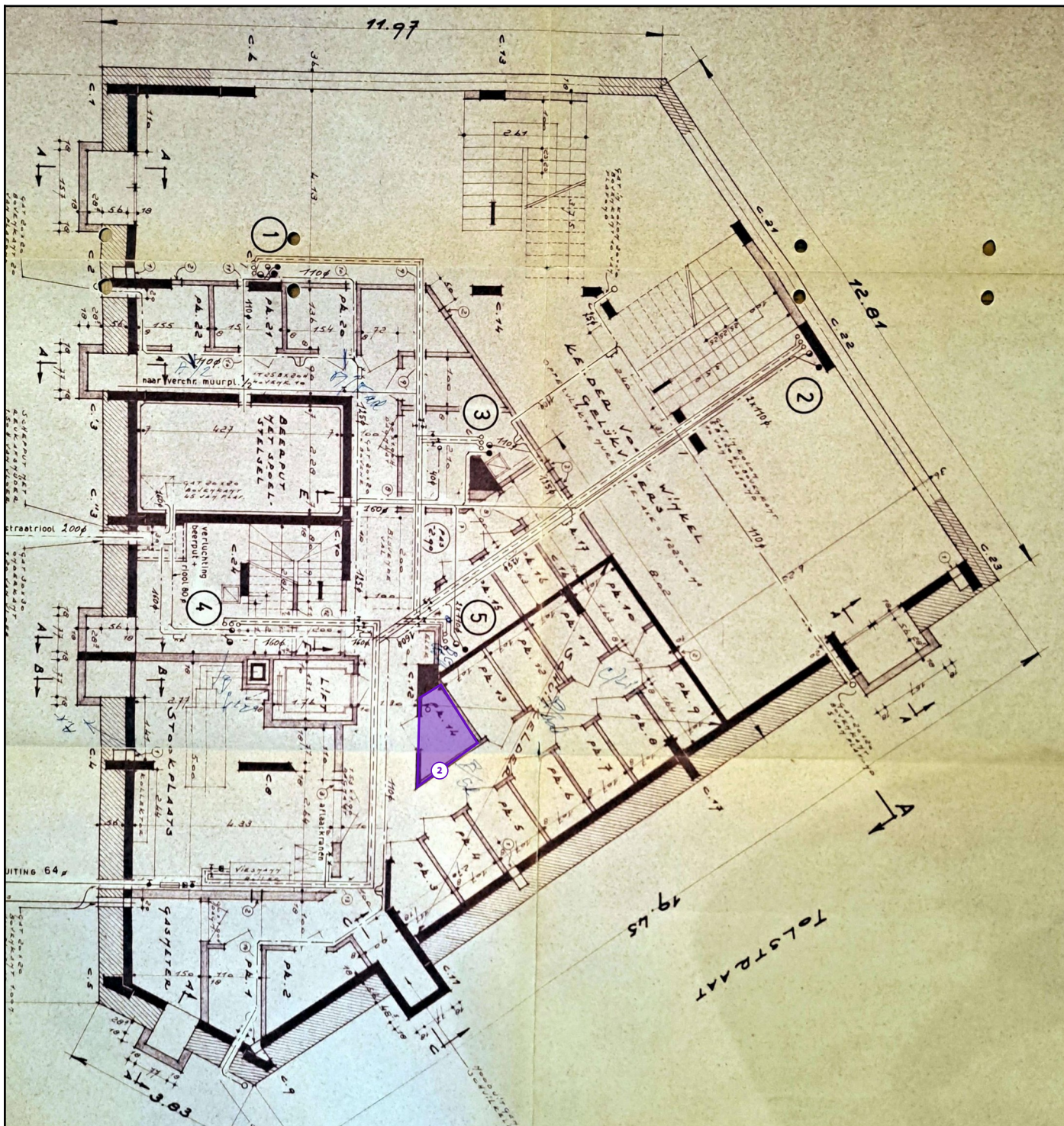
Legende van plan 2.1: Plan kelder
