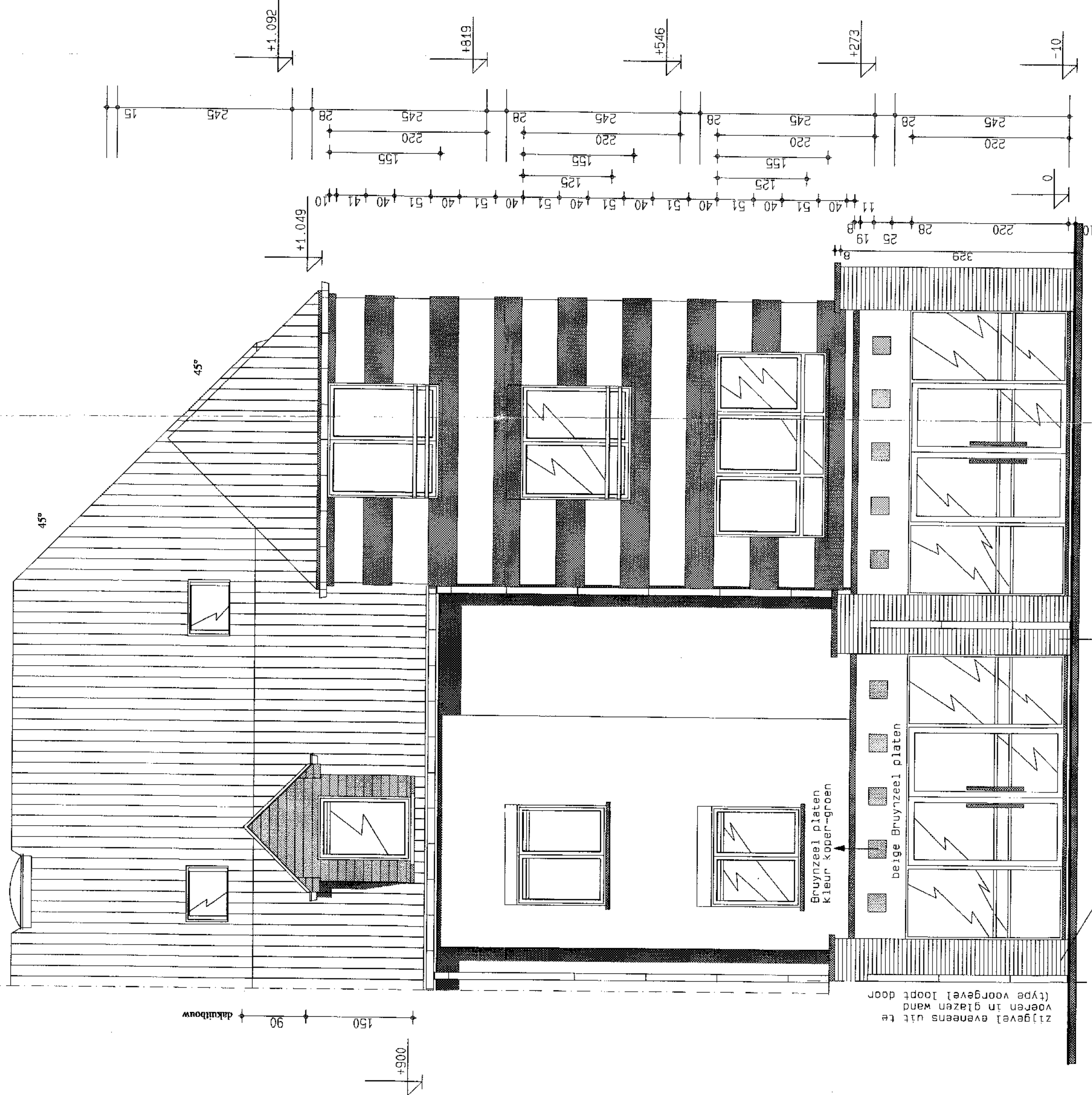
Gevelaanzicht Kapellestraat
