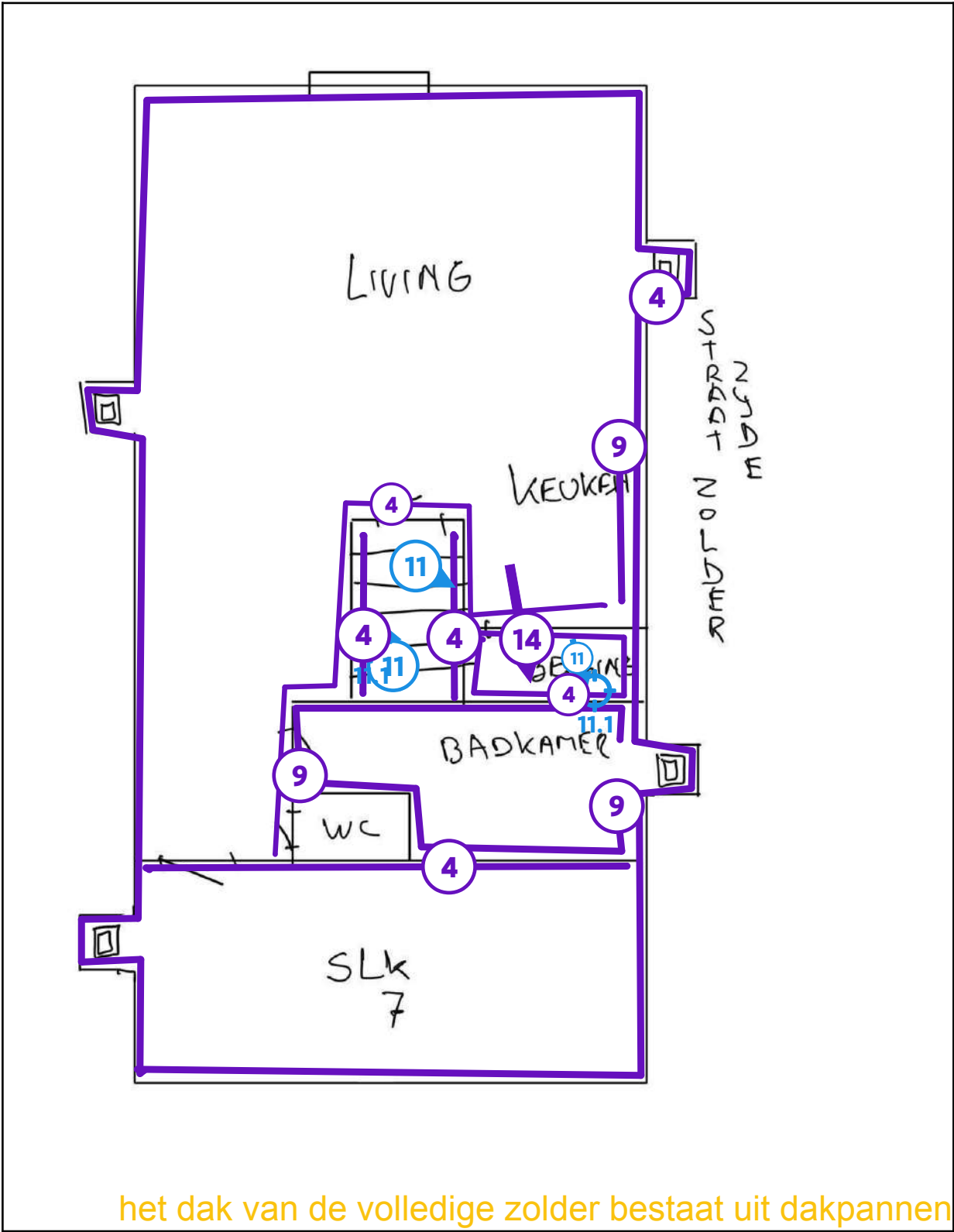
Legende van plan 1.17: Zolderstudio kopie kopie kopie
