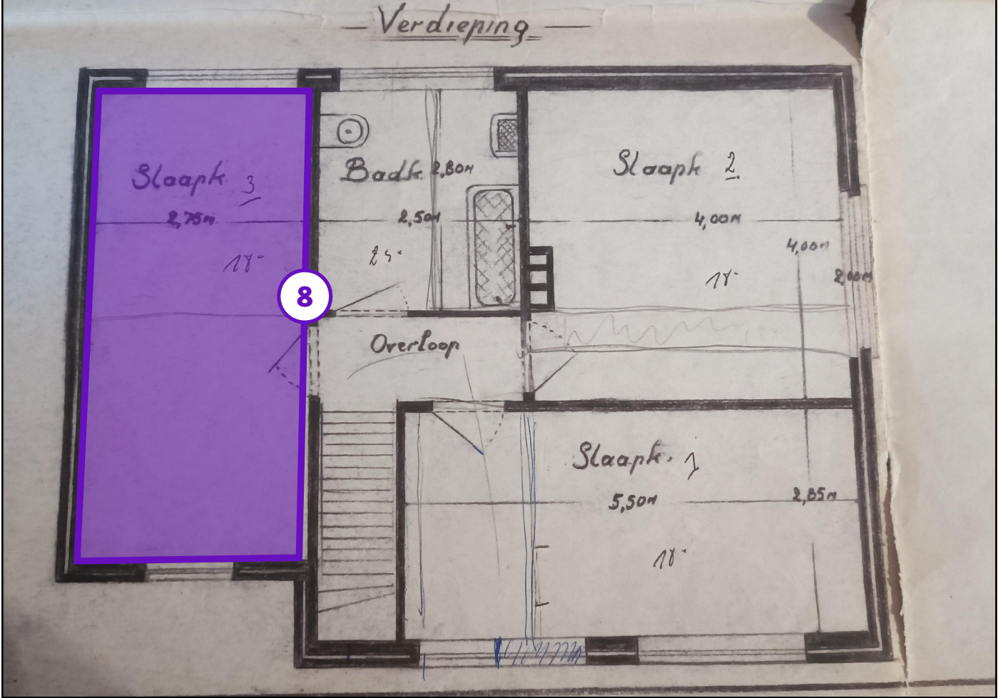
Legende van plan 1.2: Eerste verdieping
