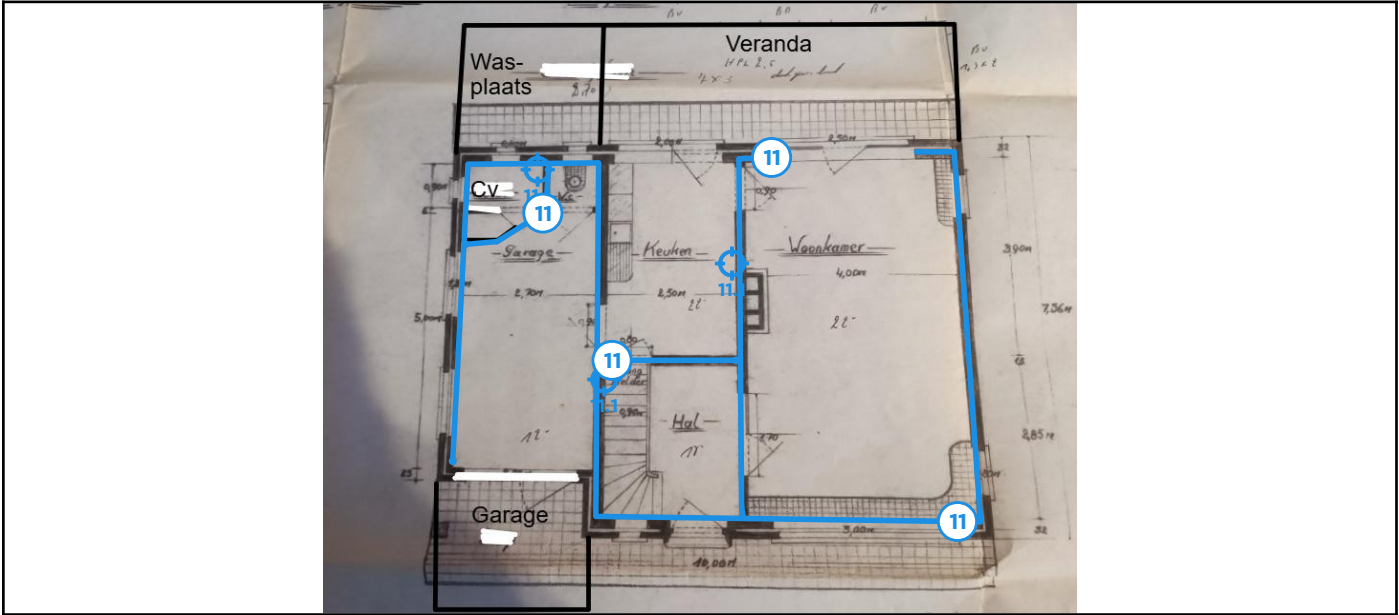
Legende van plan 1.8: Gelijkvloers
