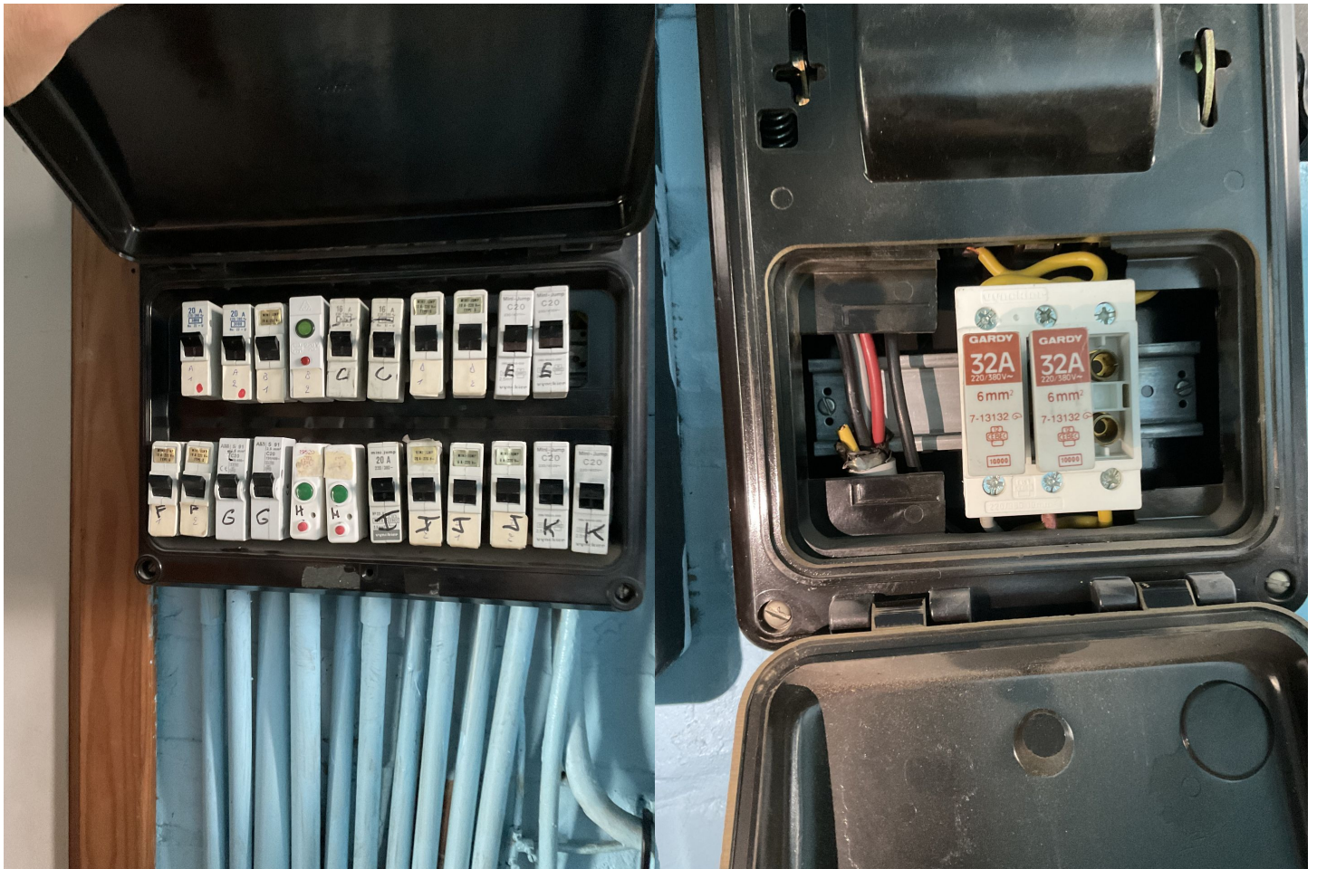
Verdeelbord 1
