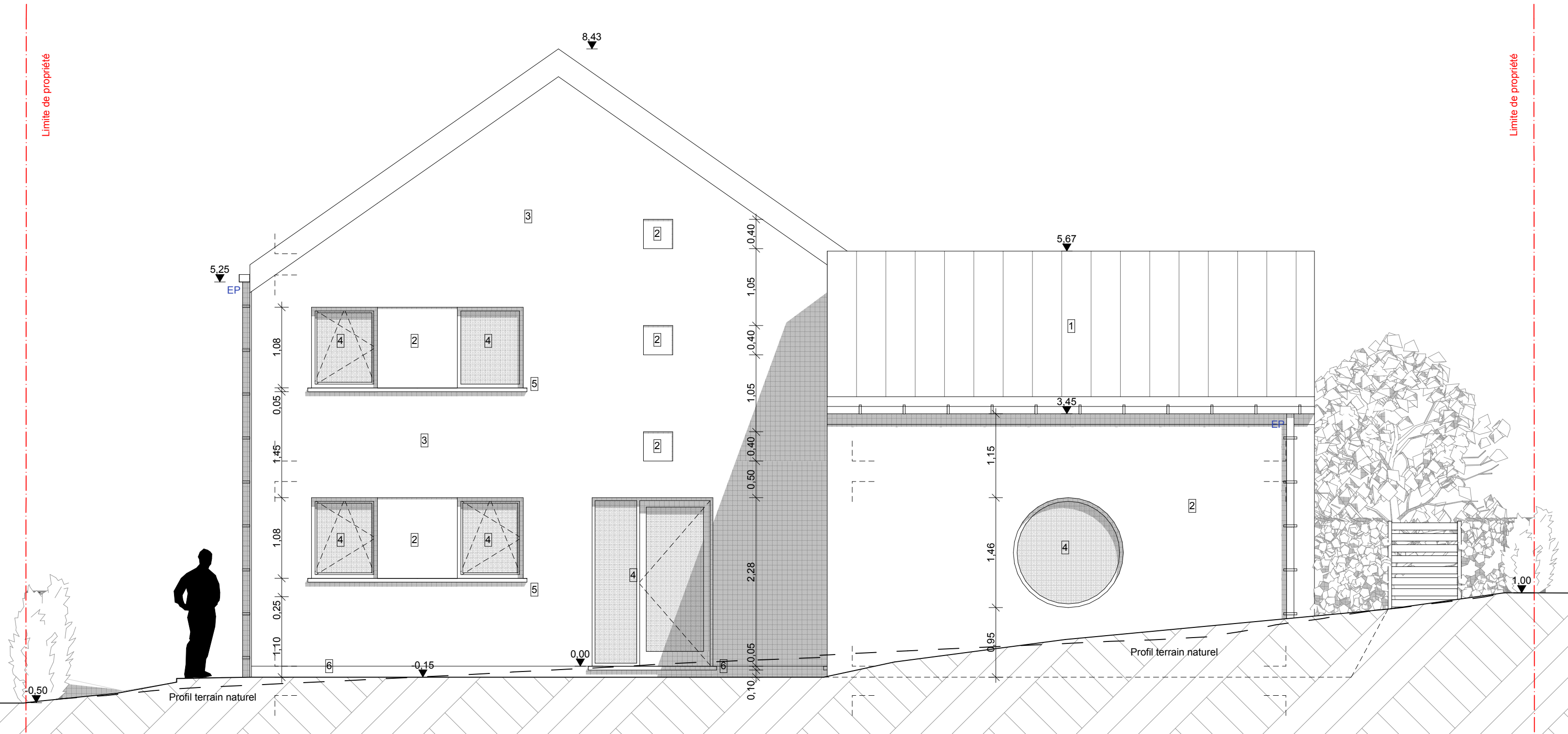
Façade avant
