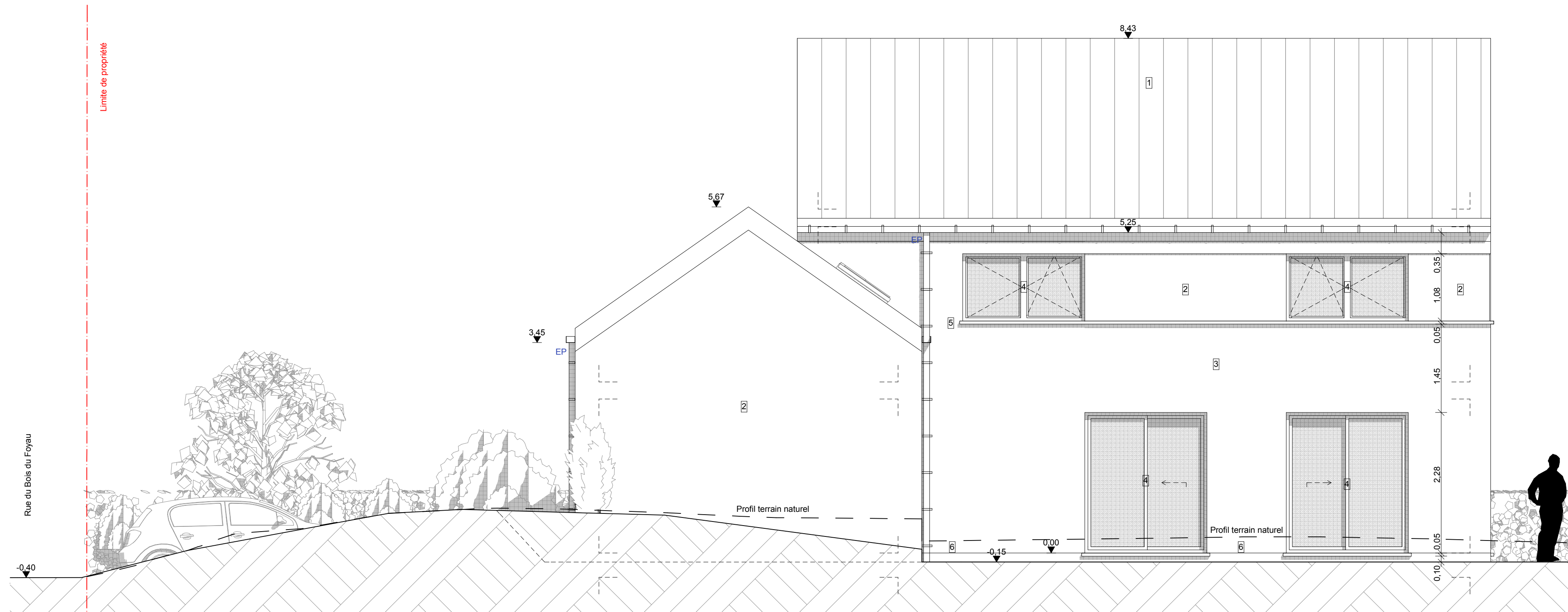
Façade droite
