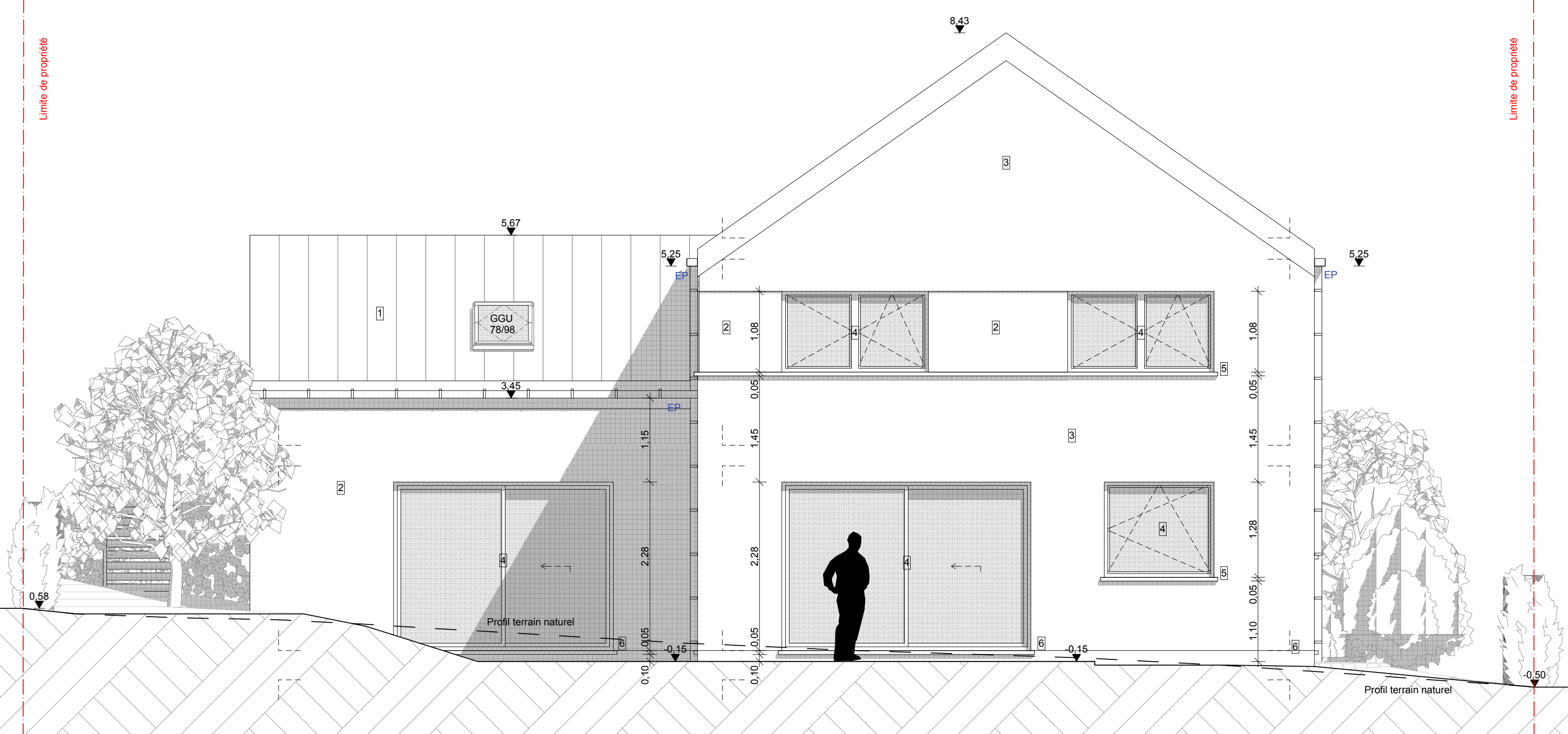
Façade arrière
