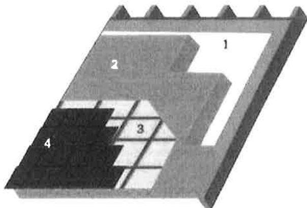
1. Dampscherf | 2. Isolatie | 3. Onderdak | 4. Dakbekleding
