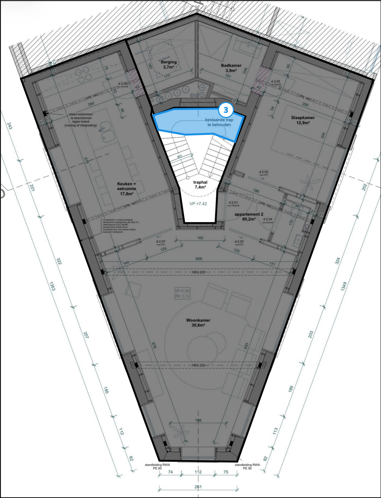
Legende van plan 1.4: Plan verdiep +2
