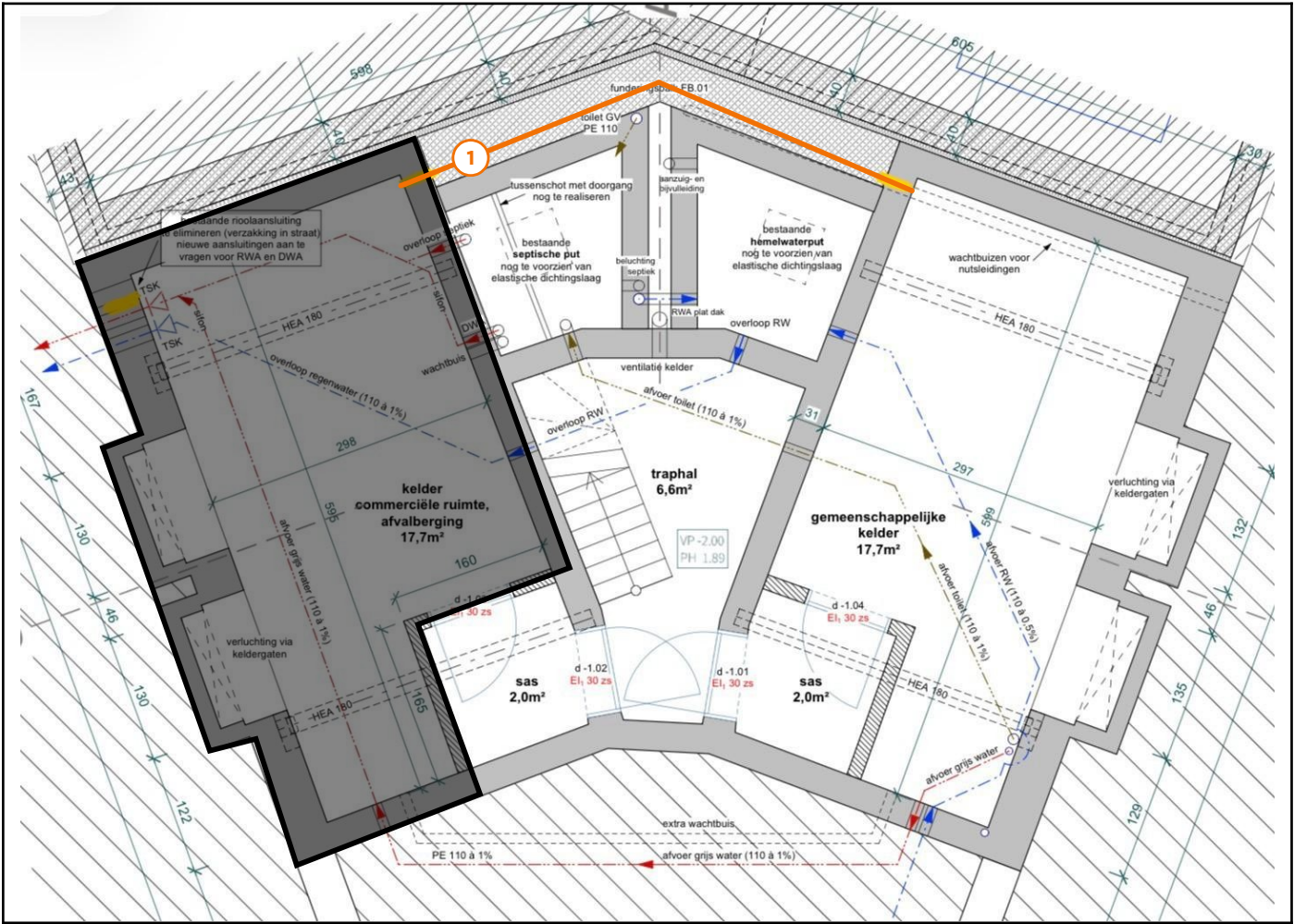
Legende van plan 1.1: Plan kelder
