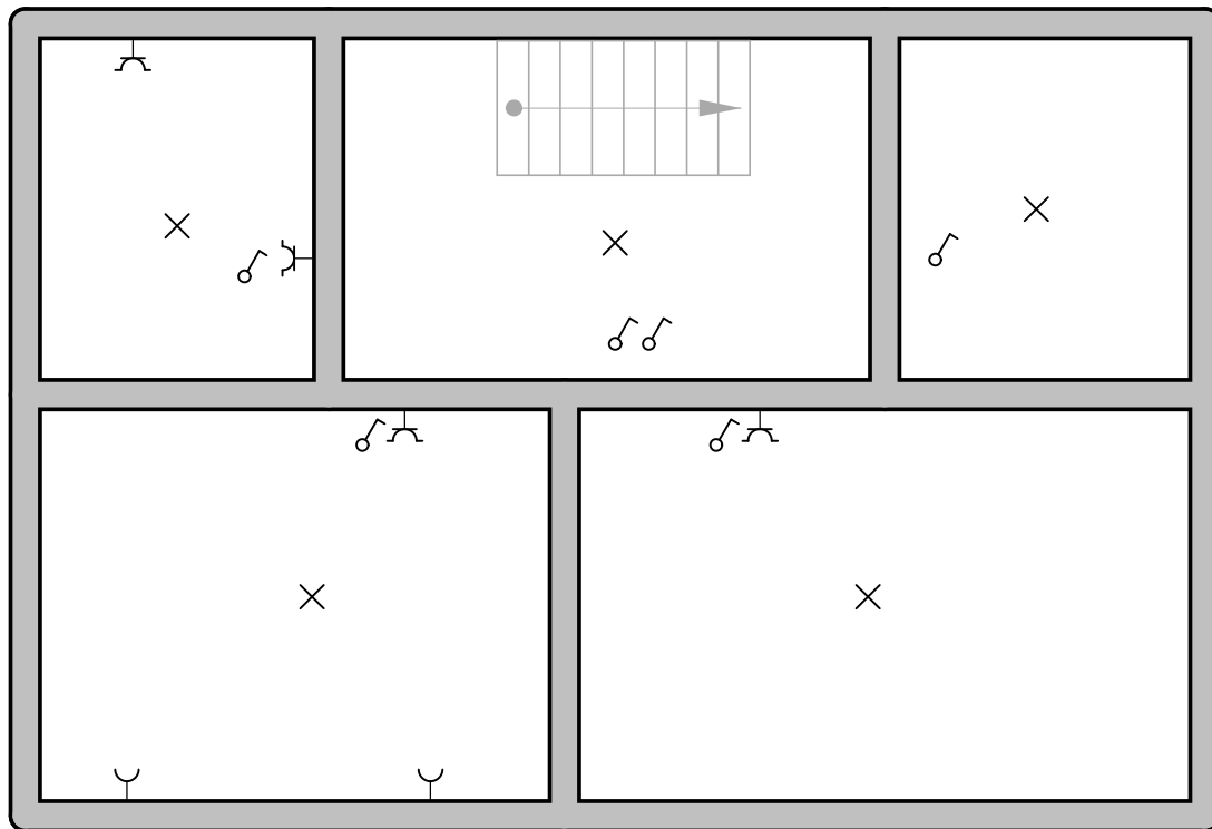
1e Verdieping
