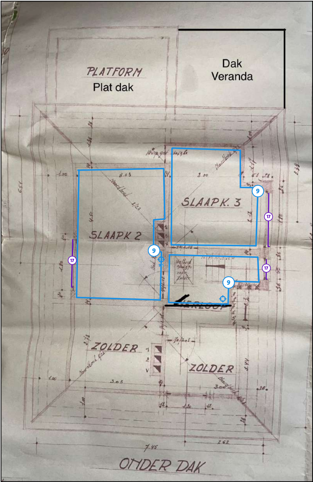
Legende van plan 1.5: 1 ste verdieping
