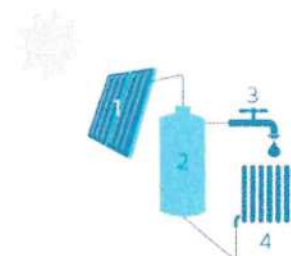
1 Zonnecollector | 2 Opslagvat voor boiler | 3 Sanitair warm water | 4 Afgifte-element voor ruimteverwarming (opdroger)
