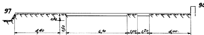
DOORSNEDE 89-89
