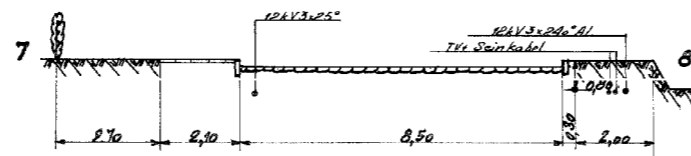
DOORSNEDE 58-58
