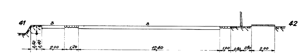
DOORSNEDE 21-21
