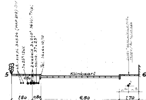
DOORSNEDE 105-105
