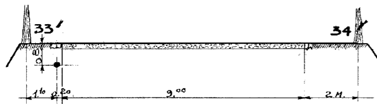
DOORSNEDE 122 122
