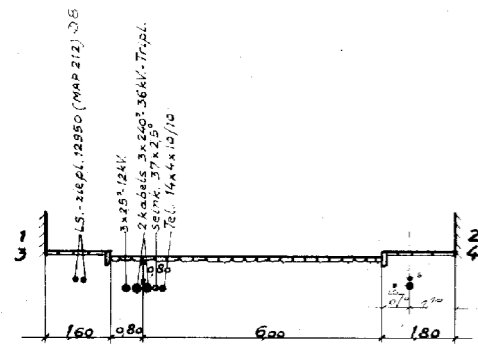
DOORSNEDE 104-104
