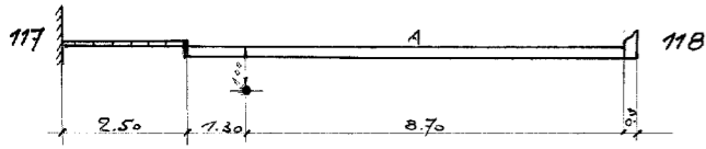
DOORSNEDE 98-98
