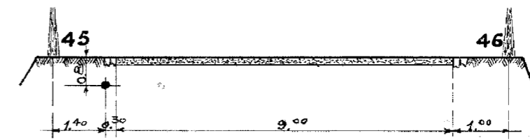
DOORSNEDE 116-116
