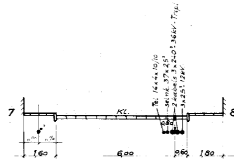
DOORSNEDE 106-106
