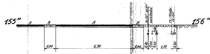
DOORSNEDE 51-51
