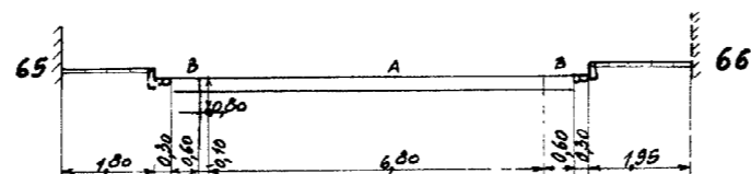
DOORSNEDE 33-33
