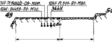
DOORSNEDE 64-64
