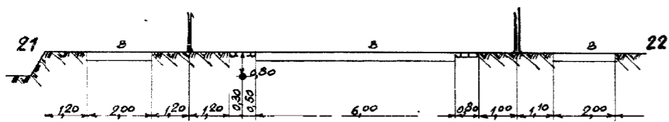
DOORSNEDE 11-11
