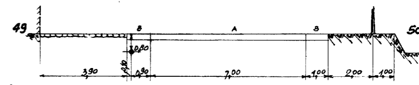
DOORSNEDE 25-25
