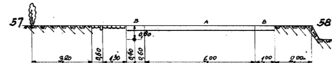
DOORSNEDE 69-69
