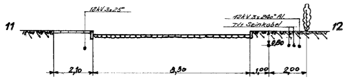
DOORSNEDE 60-60
