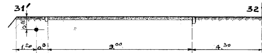
DOORSNEDE 123 123
