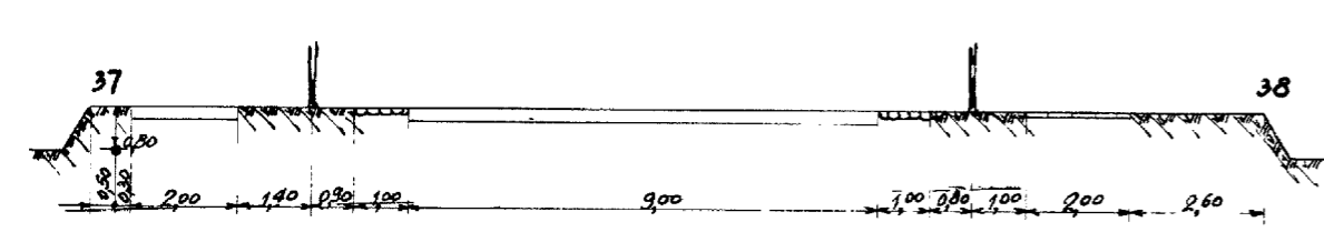
DOORSNEDE 19-19
