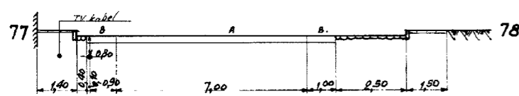
DOORSNEDE 39-39
