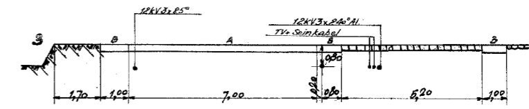
DOORSNEDE 56-56
