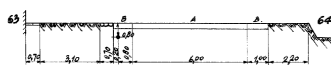
DOORSNEDE 72-72
