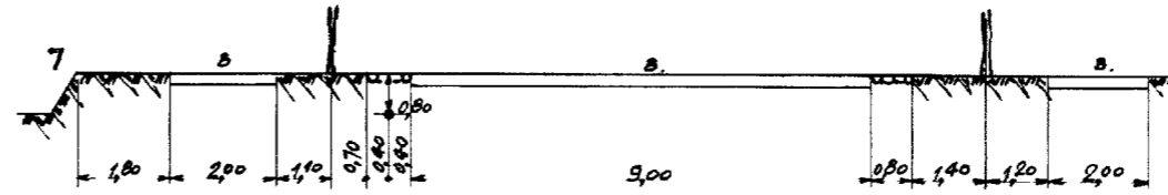
DOORSNEDE 4-4
