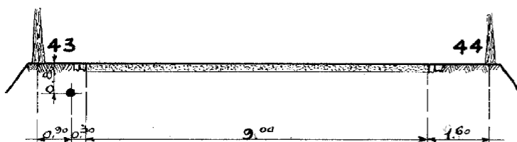
DOORSNEDE 117-117
