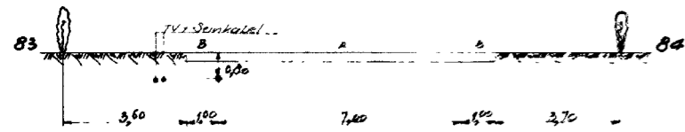
DOORSNEDDE 12-12
