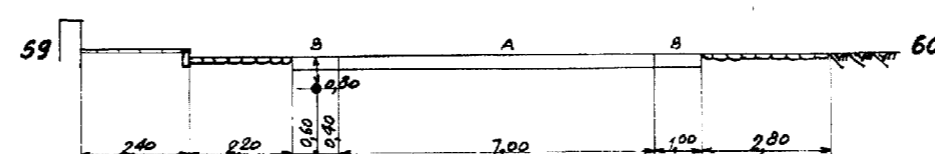
DOORSNEDE 30-30
