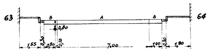
DOORSNEDE 32-32
