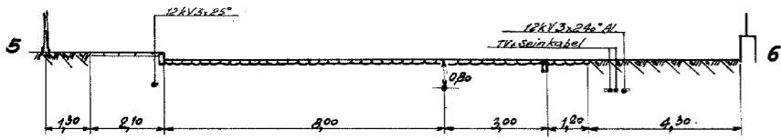
DOORSNEDE 57-57
