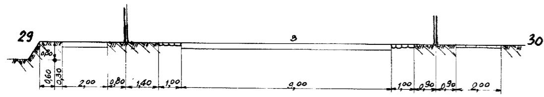
DOORSNEDE 15-15
