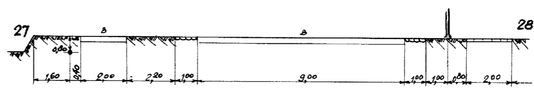
DOORSNEDE 14-14
