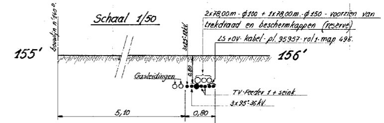
DOORSNEDE 50-50
