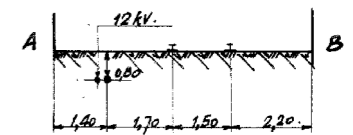
DOORSNEDE 70-70
