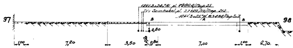
DOORSNEDE 51-51
