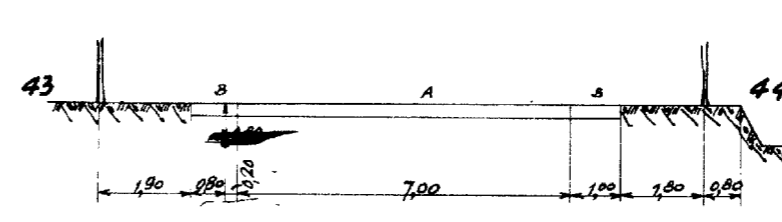
DOORSNEDE 22-22
