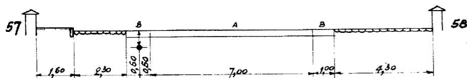
DOORSNEDE 29-29
