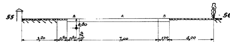
DOORSNEDE 28-28
