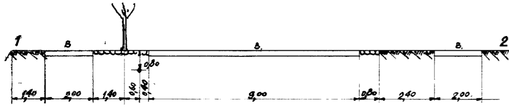
DOORSNEDE 1-1
