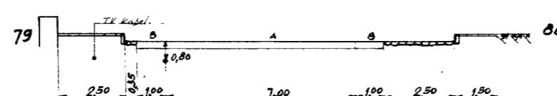
DOORSNEDE 40-40
