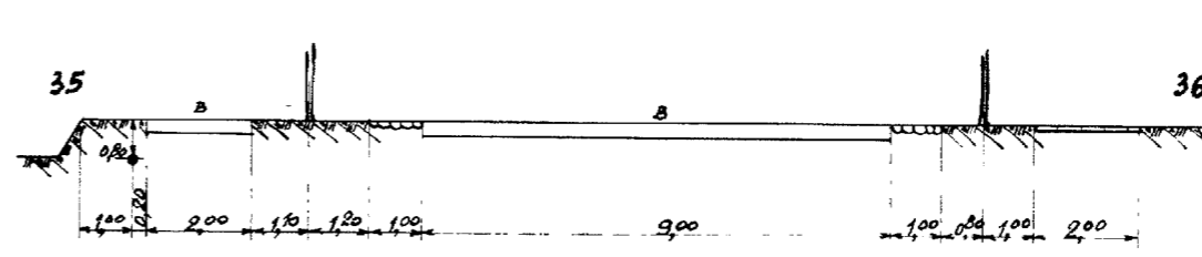
DOORSNEDE 18-18
