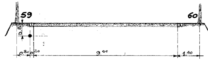
DOORSNEDE 109-109
