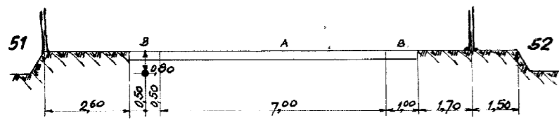
DOORSNEDE 26-26
