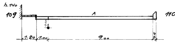
DOORSNEDE 94-94
