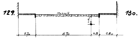
DOORSNEDE 121-101
