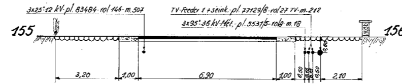
DOORSNEDE 49-49
