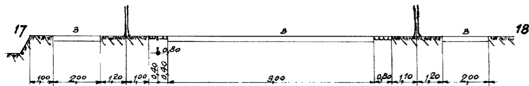
DOORSNEDE 9-9
