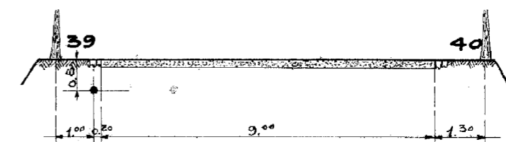
DOORSNEDE 119-119
