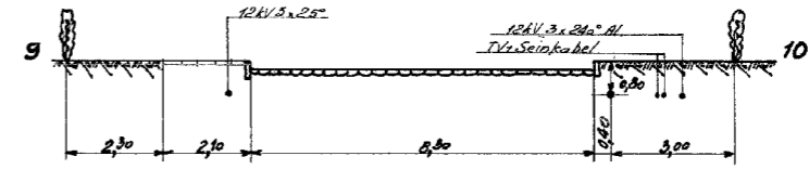
DOORSNEDE 59-59
