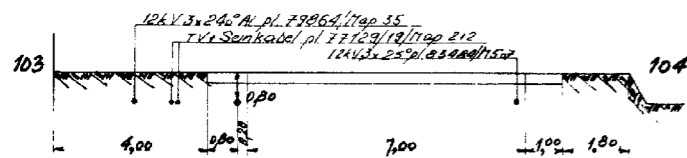
DOORSNEDE 54-54
