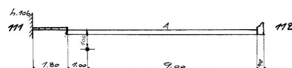
DOORSNEDE 95-95
