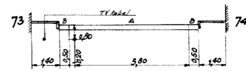
DOORSNEDE 37-37
