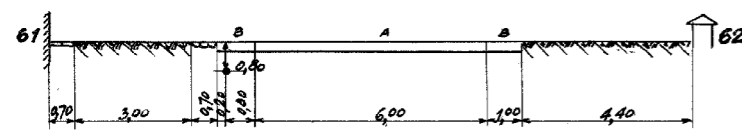
DOORSNEDE 71-71
