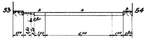
DOORSNEDE 67-67
