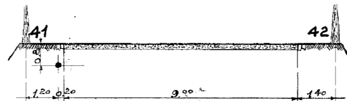
DOORSNEDE 118-118
