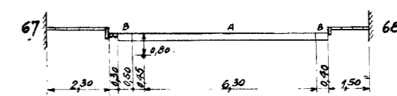
DOORSNEDE 34-34
