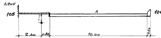
DOORSNEDE 92-92
