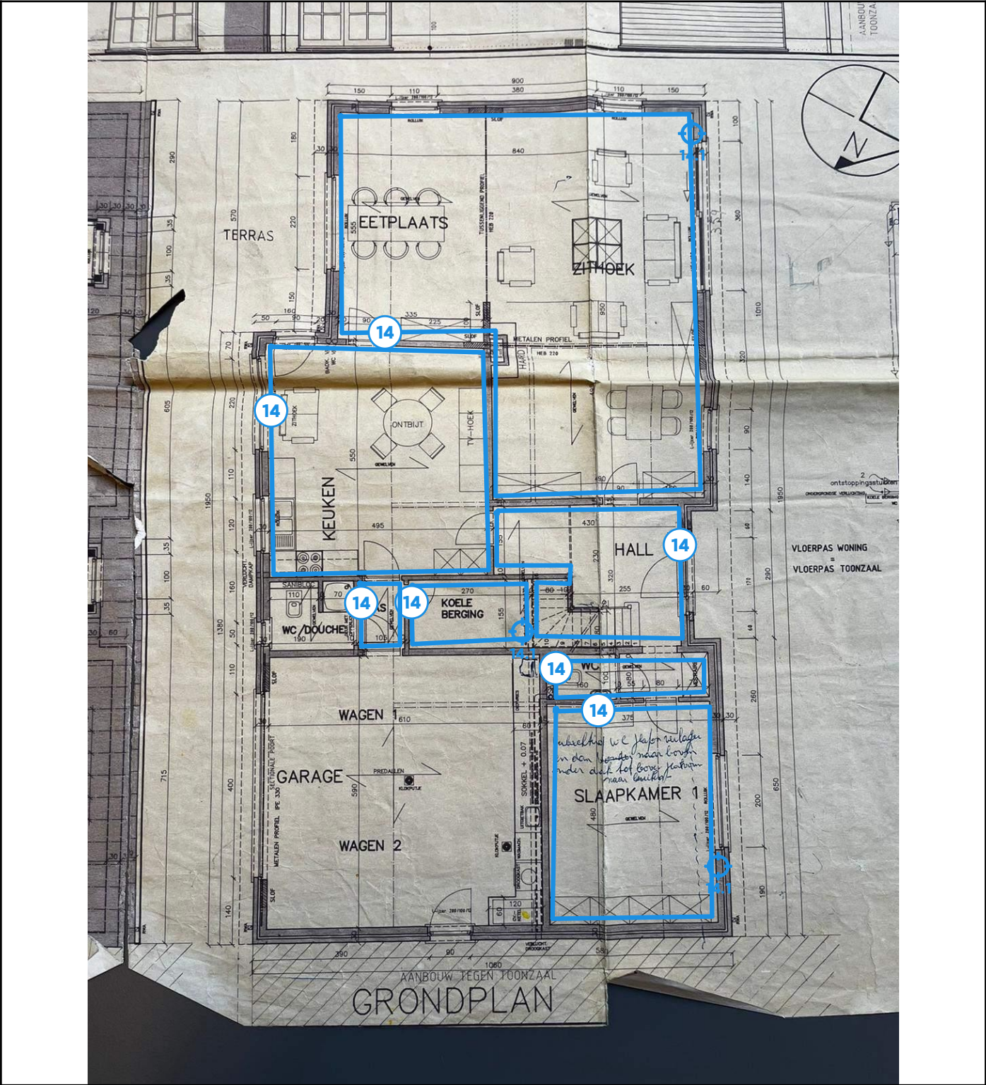
Legende van plan 1.4: Grondplan - Gelijkvloers - Muren
