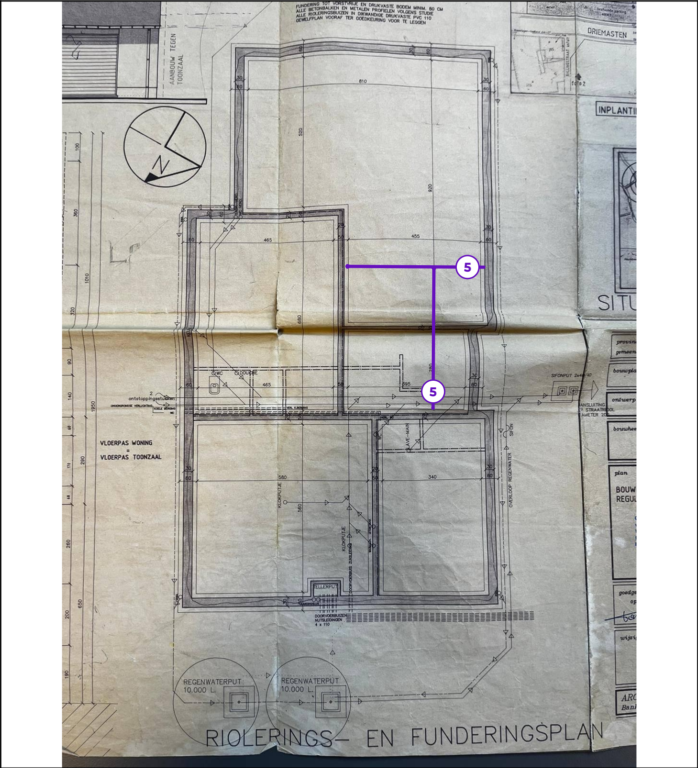
Legende van plan 1.1: Grondplan - Kelder - Kruipkelder
