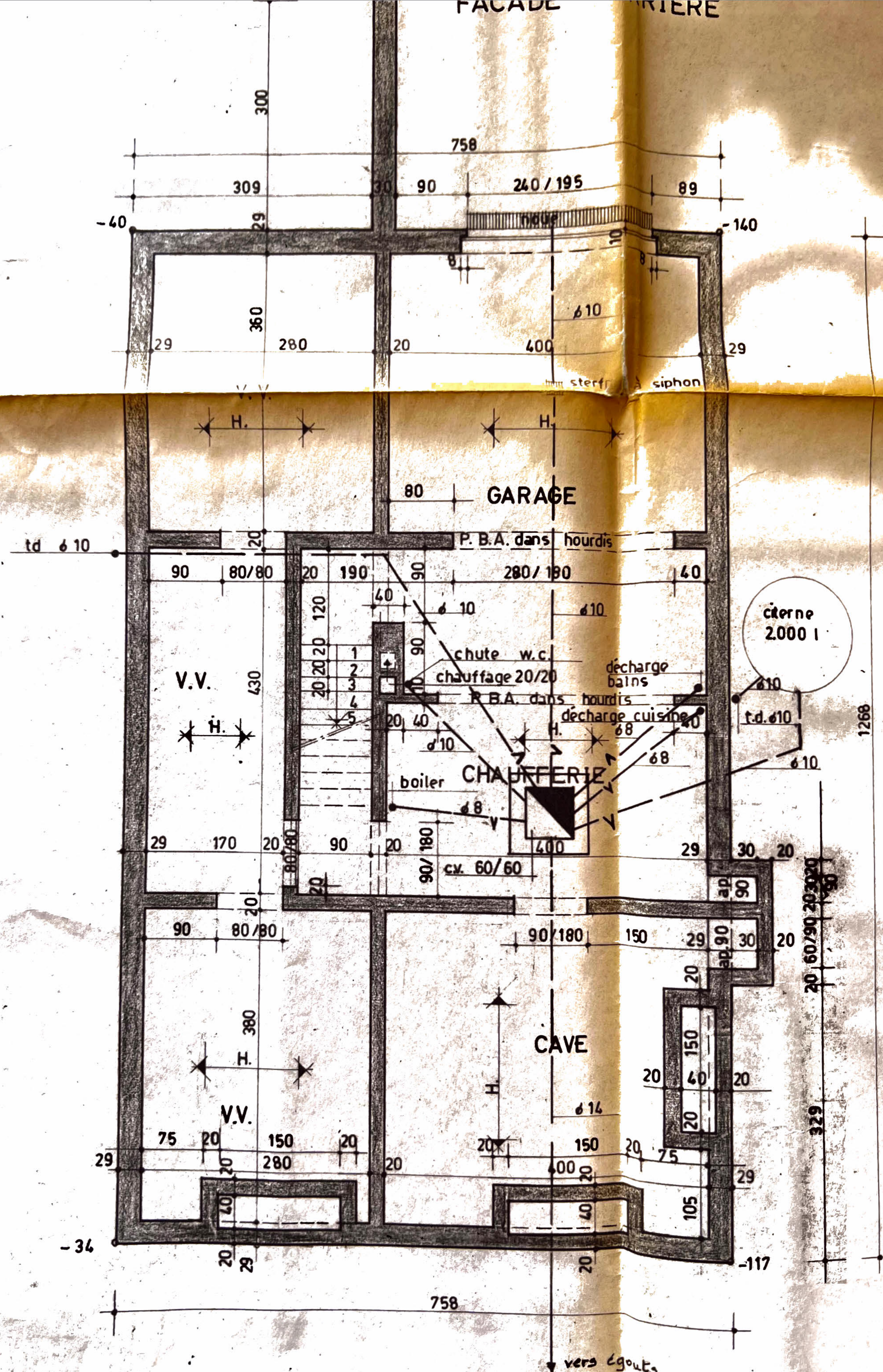
PLAN DES SOUS-SOLS
