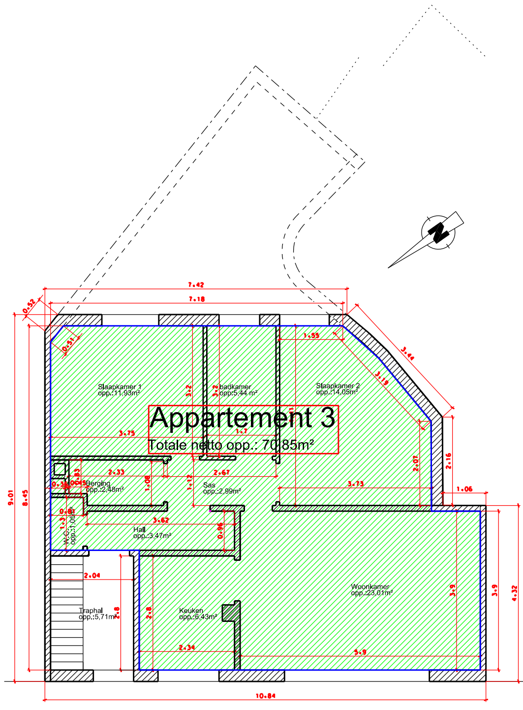
Tweede verdieping Heidebloemstraat
