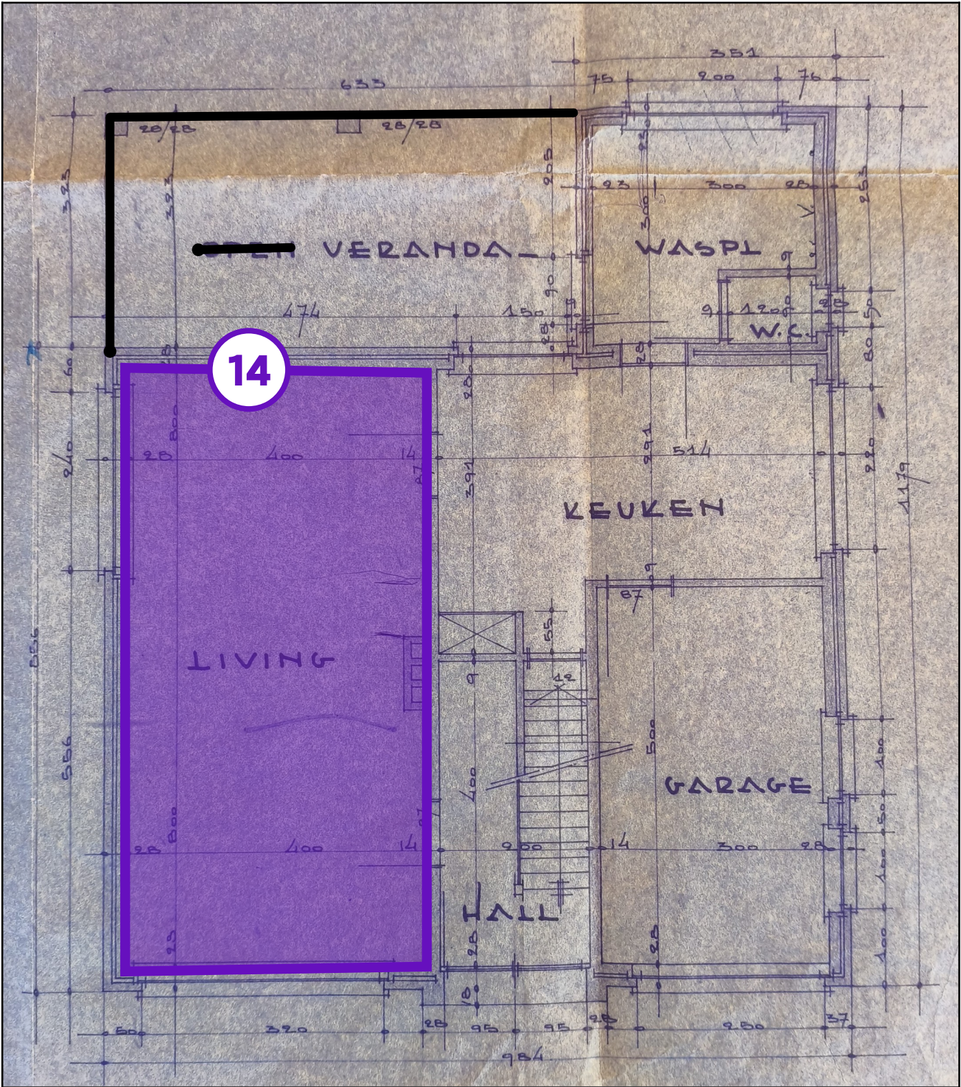
Legende van plan 1.10: Gelijkvloers
