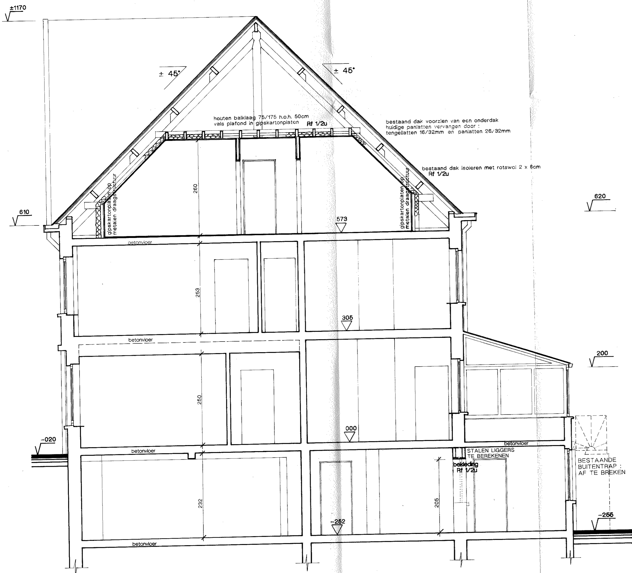
DOORSNEDE AB
