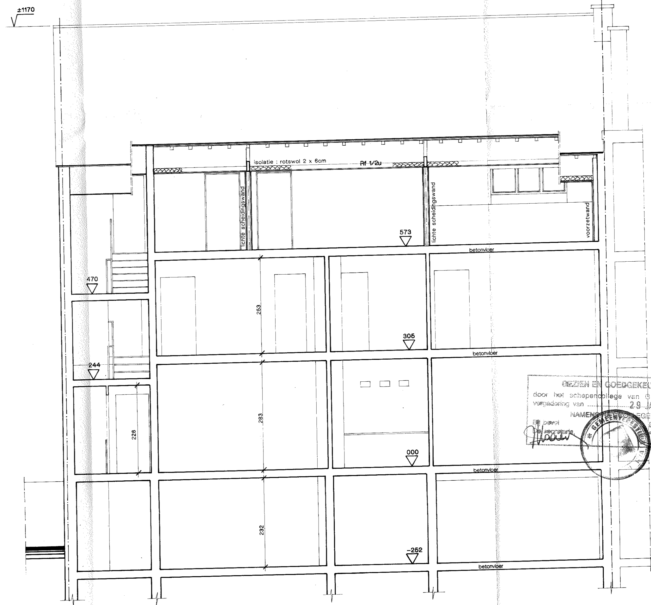
DOORSNEDE CD
