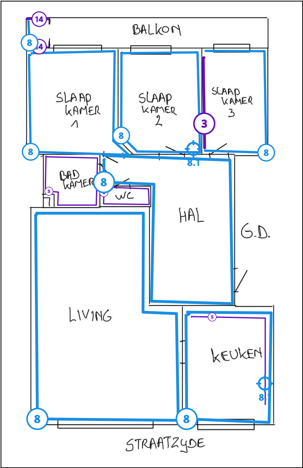
Legende van plan 1.5: Appartement
