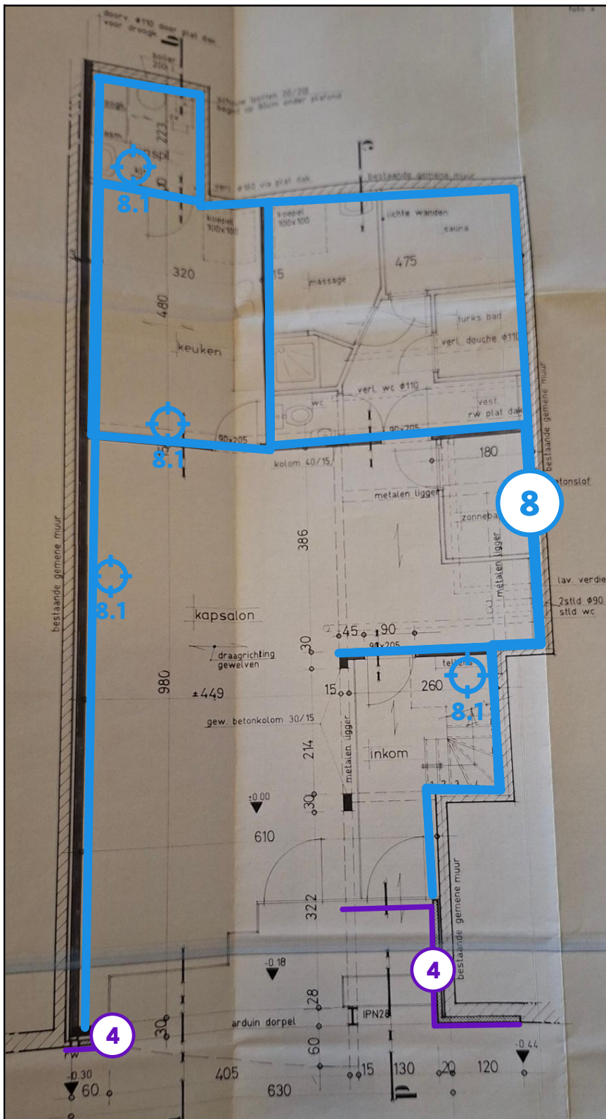
Legende van plan 1.3: grondplan gelijkvloers pleister wanden
